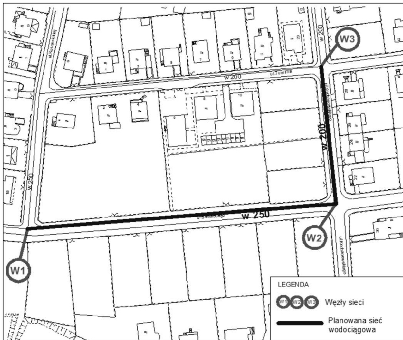
Rys. 1. Lokalizacja planowanej sieci wodociągowej – odcinki W1 – W2 i W2 – W3
