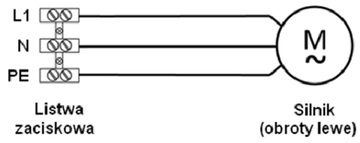
Rys 1. Schemat połączeń elektrycznych
