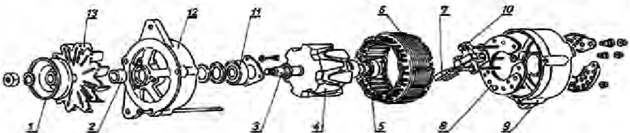
Rysunek 2. Alternator z rozłożonymi elementami.
