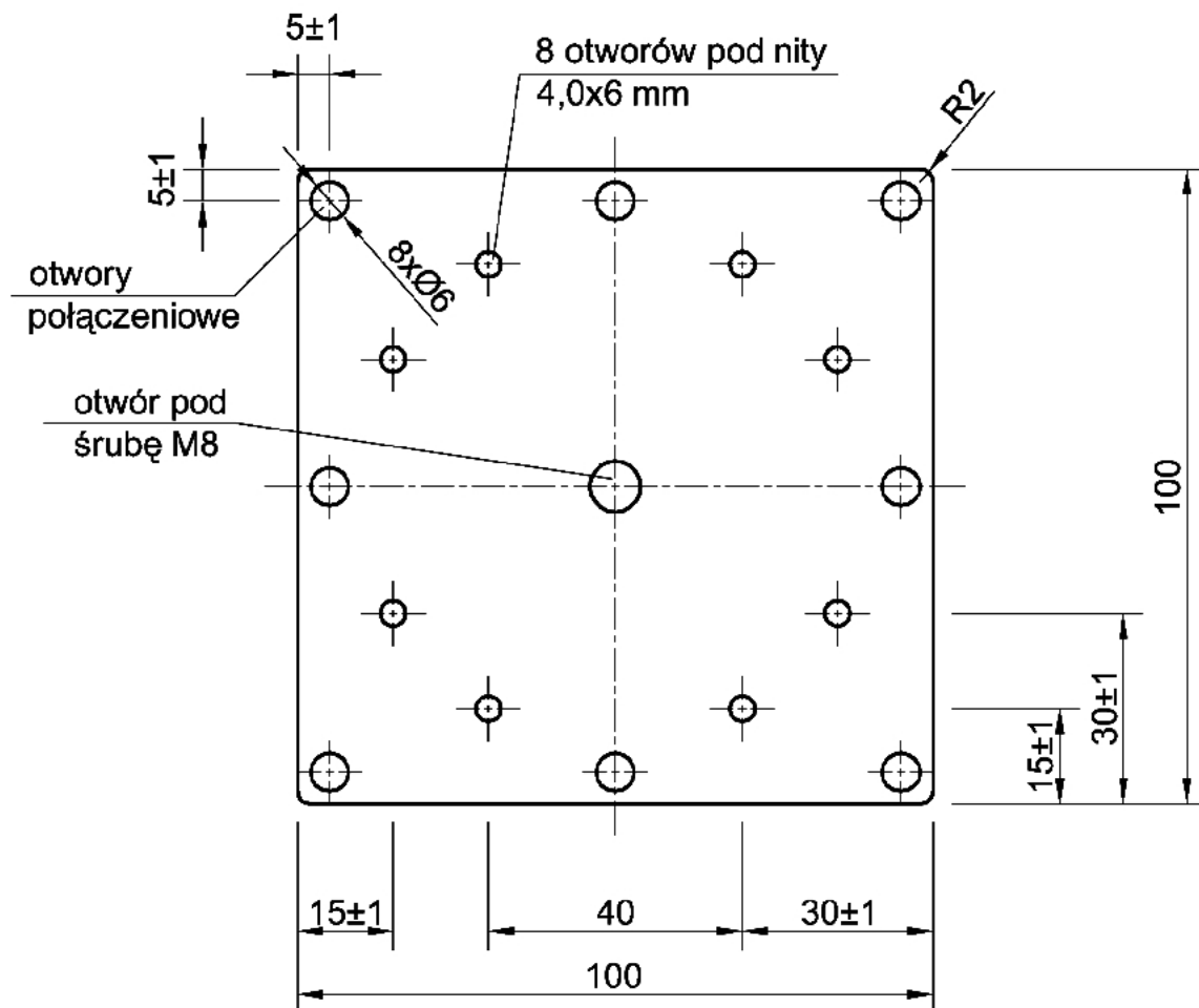
Rysunek 1. Wspornik
