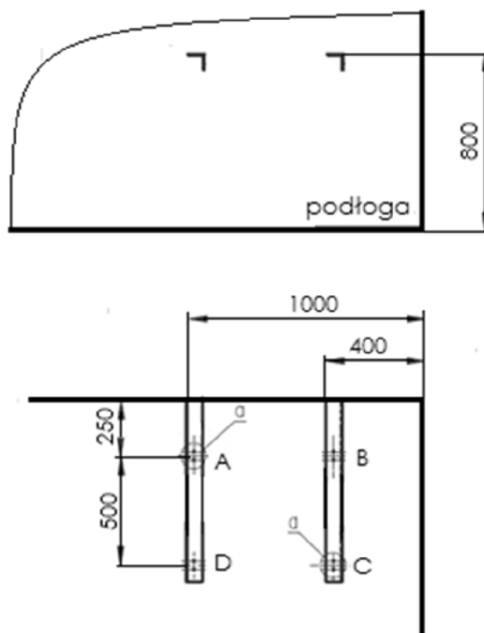
Rysunek 3. Rozmieszczenie kątowników w narożniku (wymiaru podane w mm)
