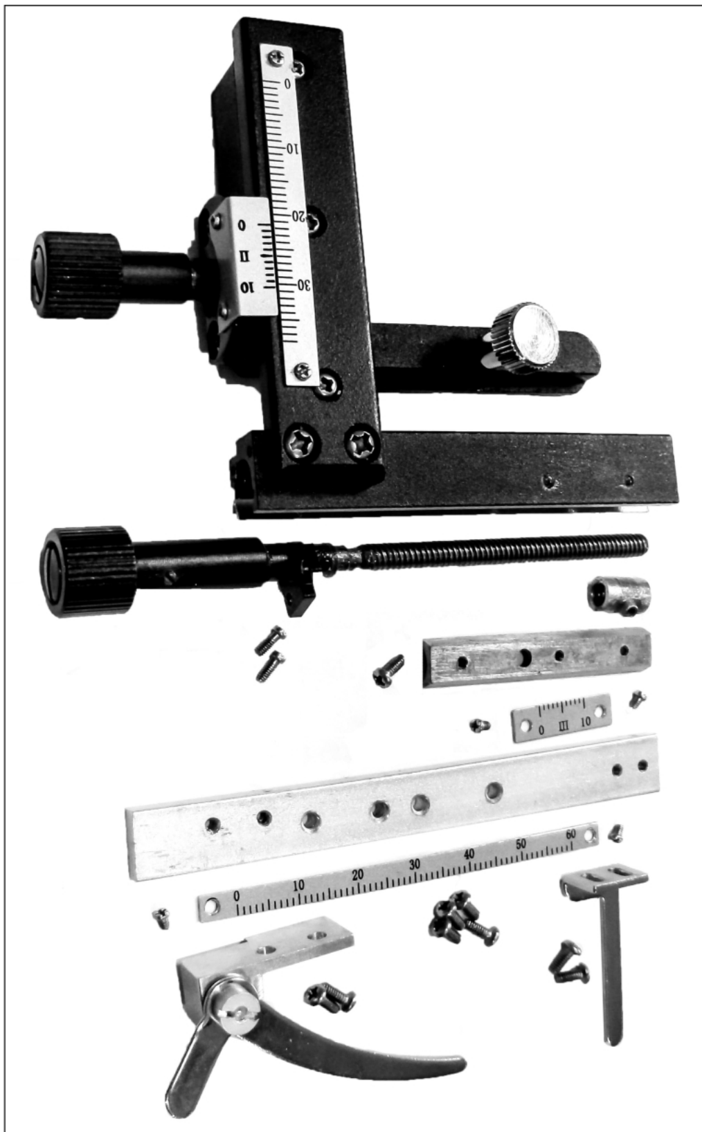
Rysunek 2. Nasadka krzyżowa do stolika mikroskopowego w rozborze na części
