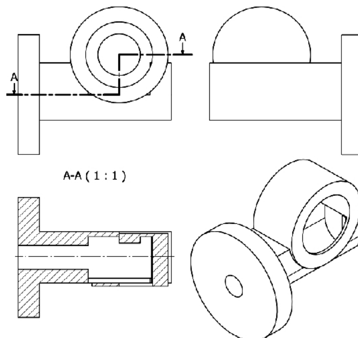
Rys. 1. Przekrój odlewu
