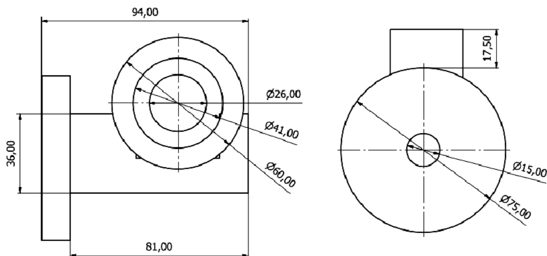
Rys. 2. Wymiary odlewu
