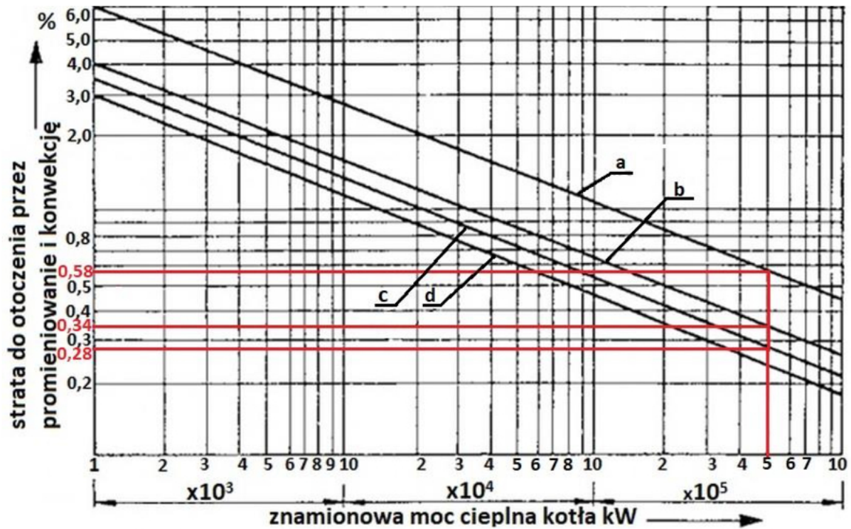
Rys. 2 Wykres zależności straty promieniowania od mocy cieplnej kotła
