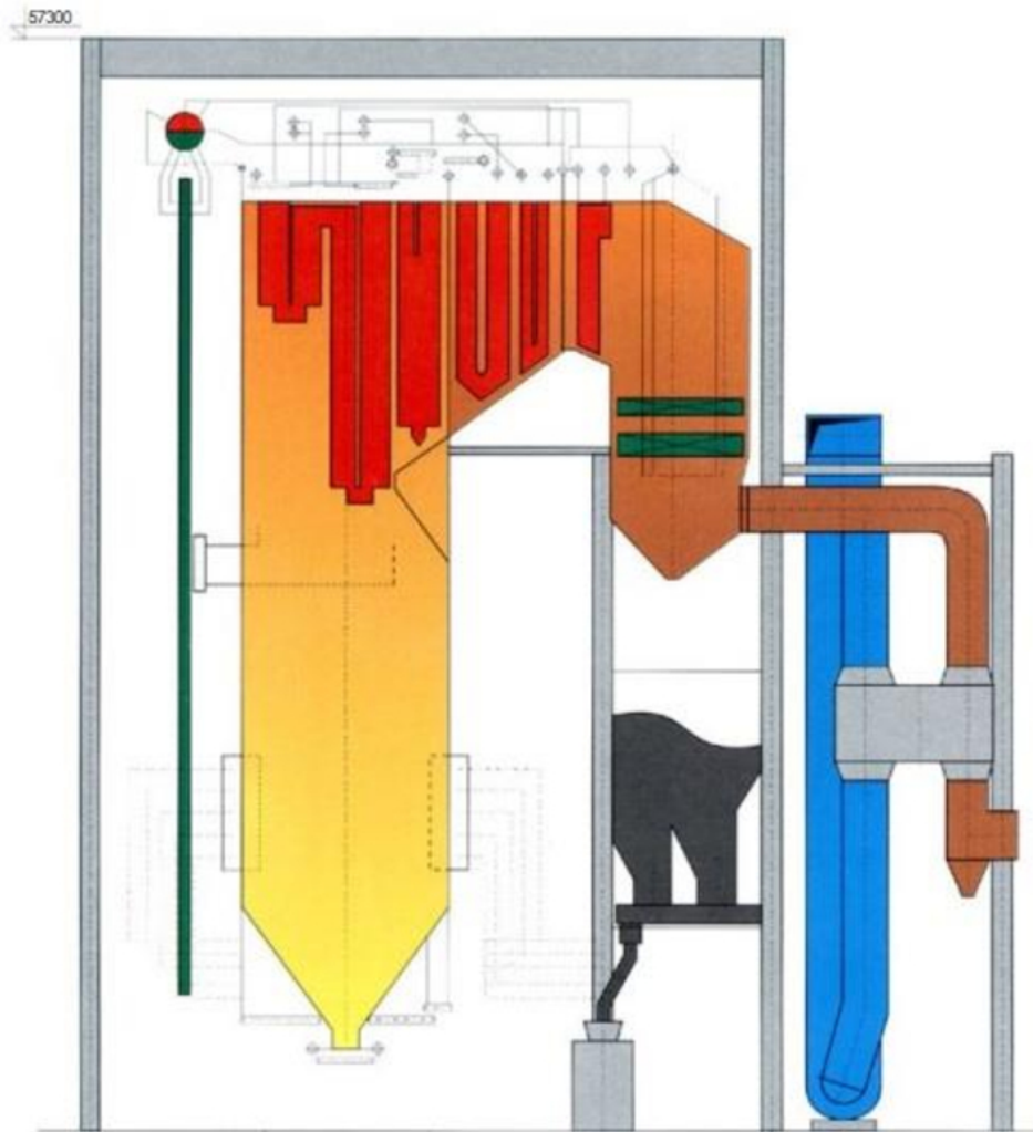
Rys. 1 Schemat kotła OP 650
