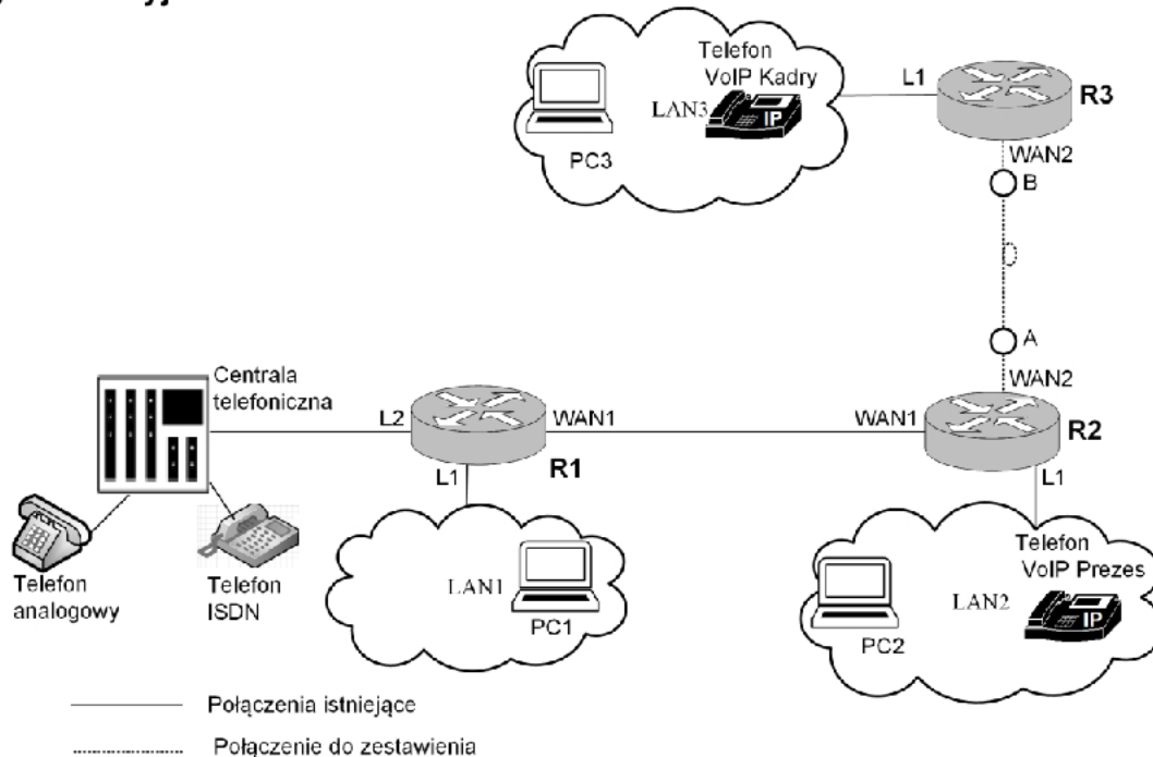
Rysunek 1. Schemat sieci telekomunikacyjnej Operatora
