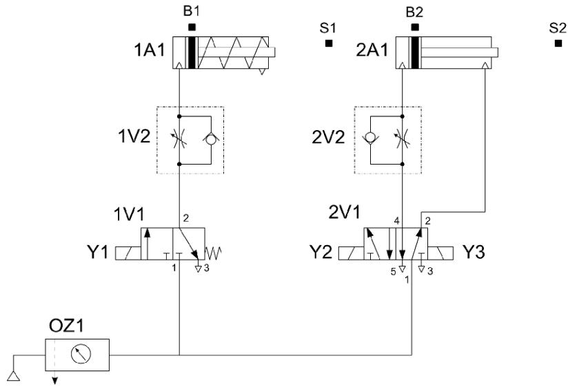
Rysunek 2. Schemat połączeń pneumatycznych układu elektropneumatycznego
