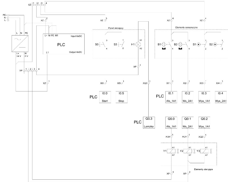
Rysunek 3. Schemat połączeń elektrycznych układu elektropneumatycznego
