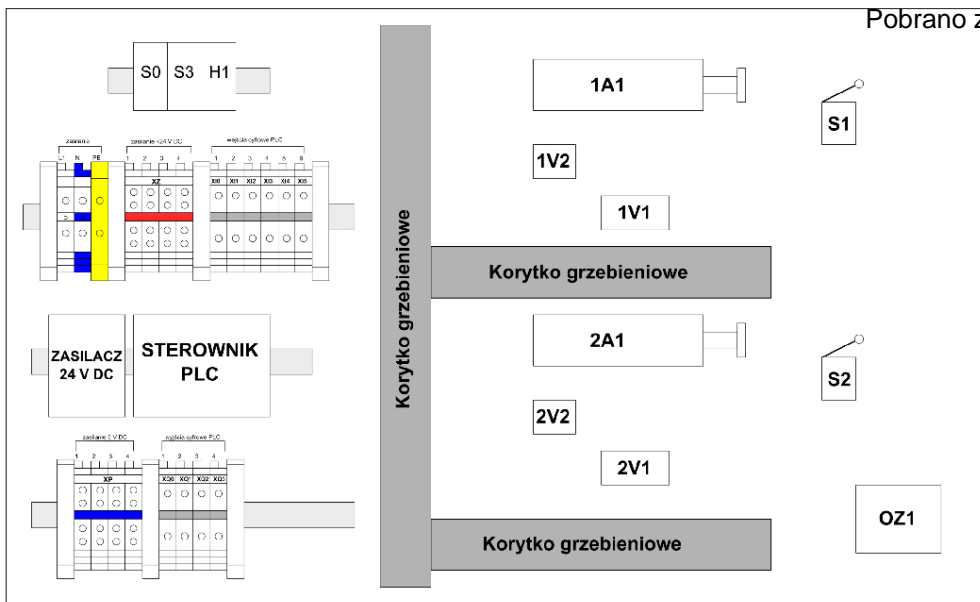
Rysunek 1. Schemat rozmieszczenia elementów układu elektropneumatycznego
