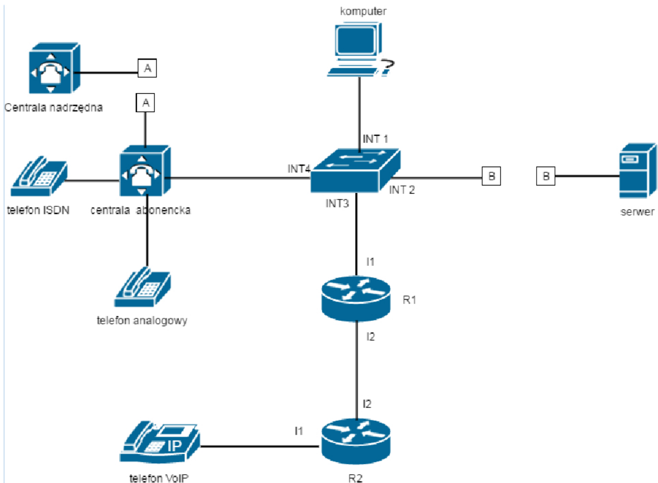
Rys. 1. Schemat usytuowania urządzeń w sieci teleinformatycznej
