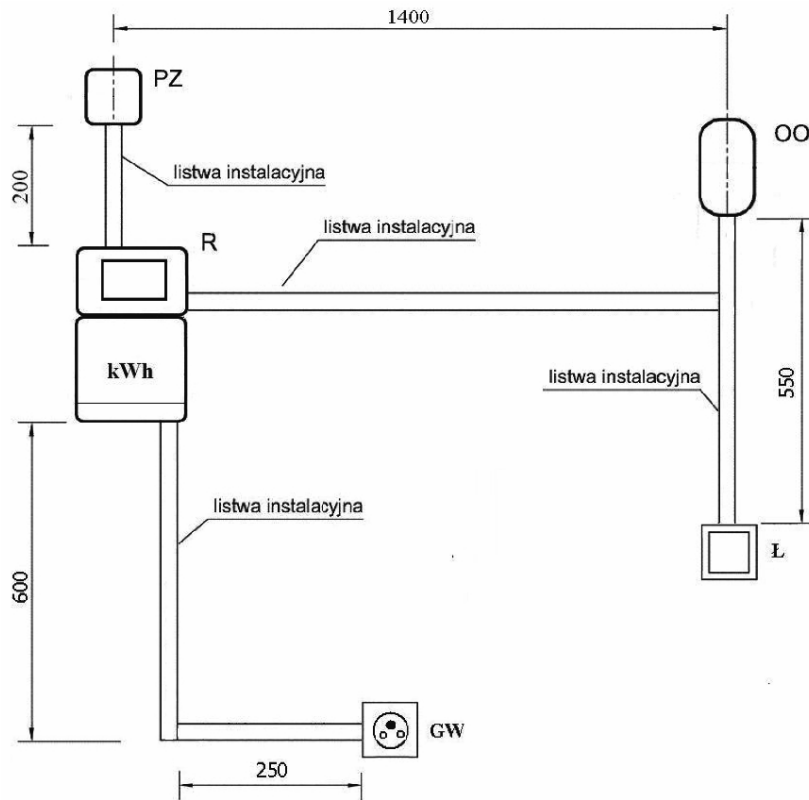
Rys. 1. Schemat rozmieszczenia elementów instalacji elektrycznej
