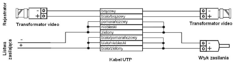
Rysunek 4. Schemat połączenia kamery z rejestratorem
