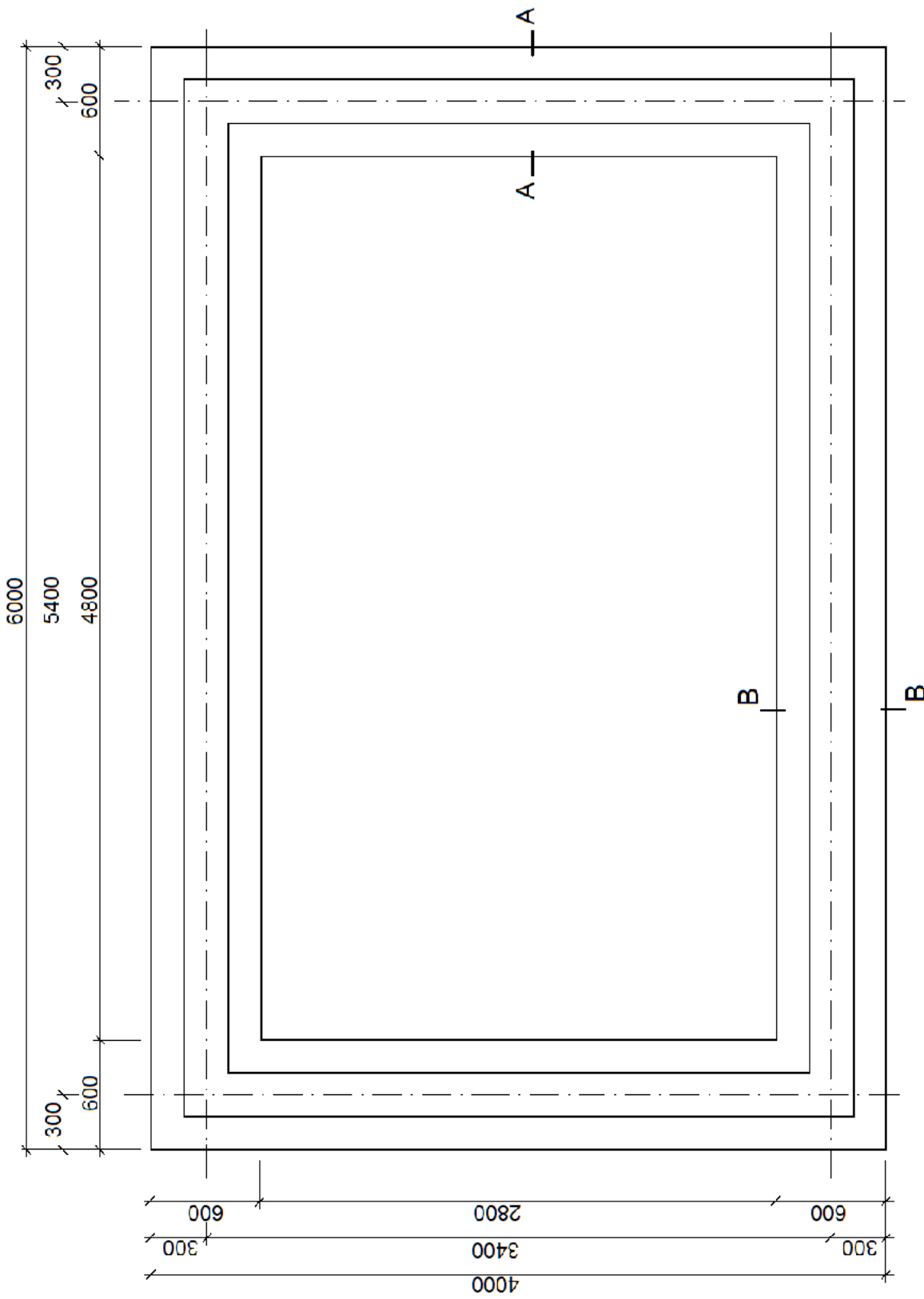
Rysunek 1. Rzut ław fundamentowych budynku zaplecza socjalnego
