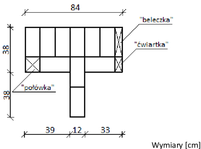
Rysunek 3. Układ cegieł w warstwach 1, 3, 5
