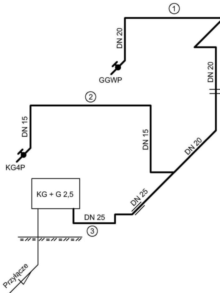
Rysunek 1. Szkic instalacji gazowej podlegającej obliczeniom projektowym
