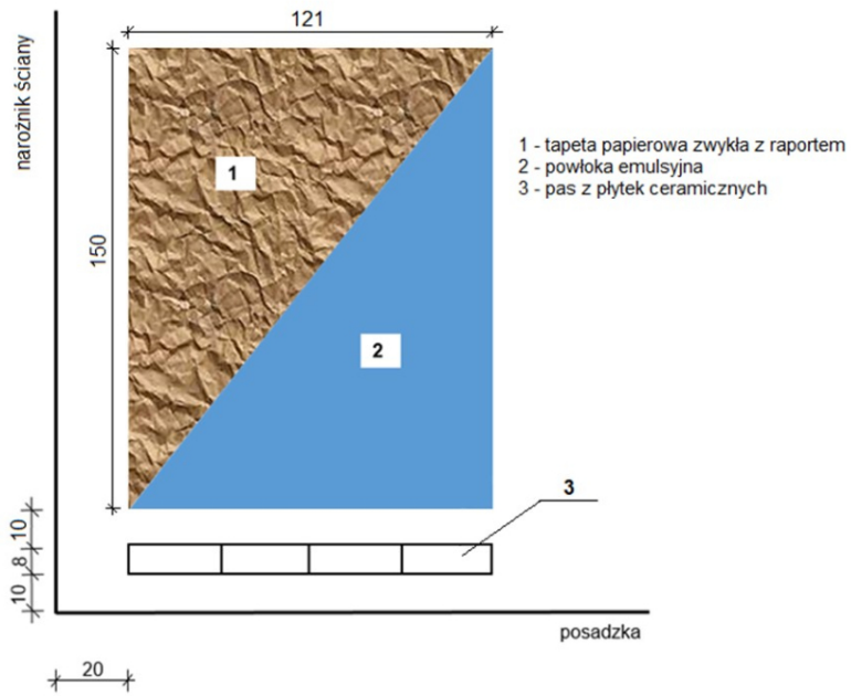
Widok ściany
