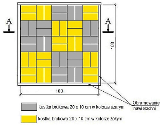
Rysunek1. Rzut poziomy fragmentu nawierzchni do ułożenia
