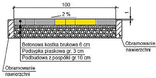
Rysunek 2. Przekrój poprzeczny nawierzchni
