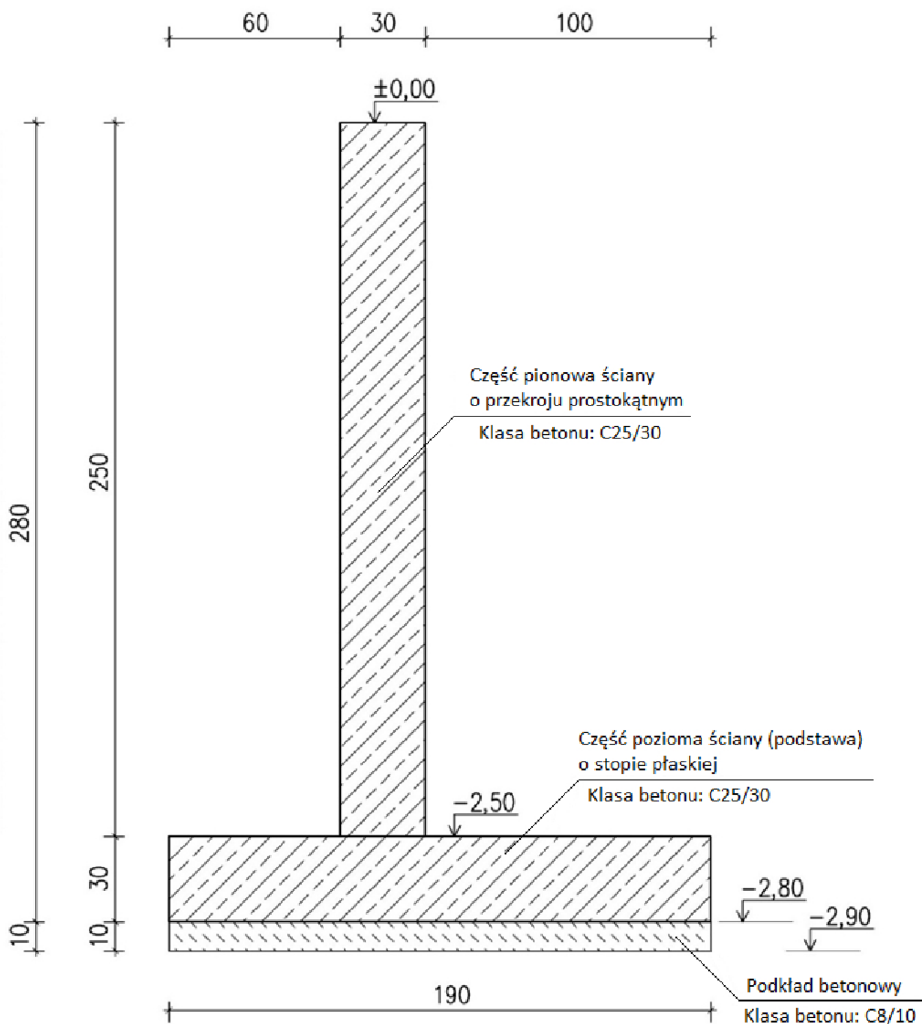
Rysunek 2. Przekrój A-A żelbetowej ściany oporowej
