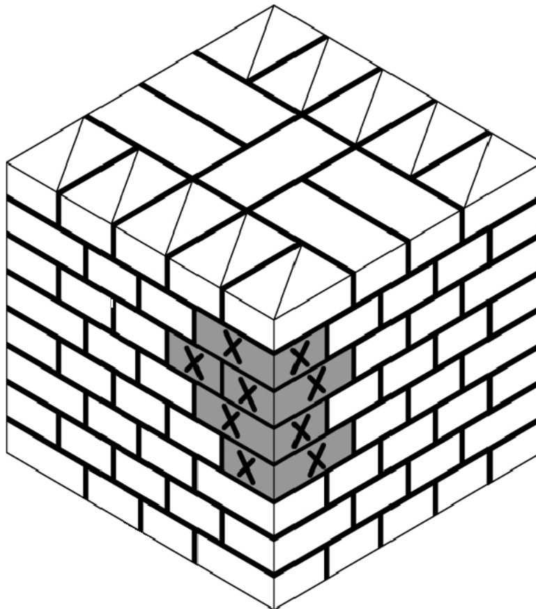
Rysunek wykonawczy
