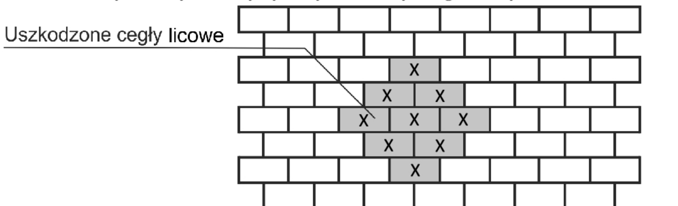
Rysunek wykonawczy wymiany uszkodzonych cegieł licowych
