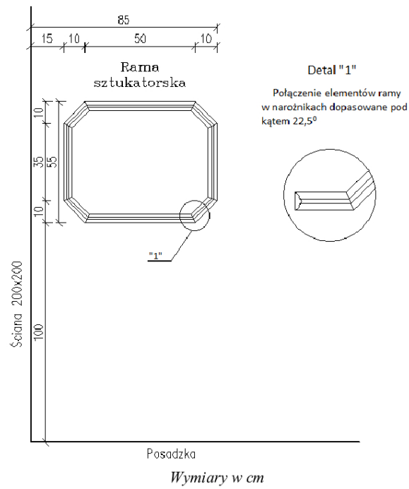
Rysunek 1. Gotowa rama sztukatorska ze ściennych profili
