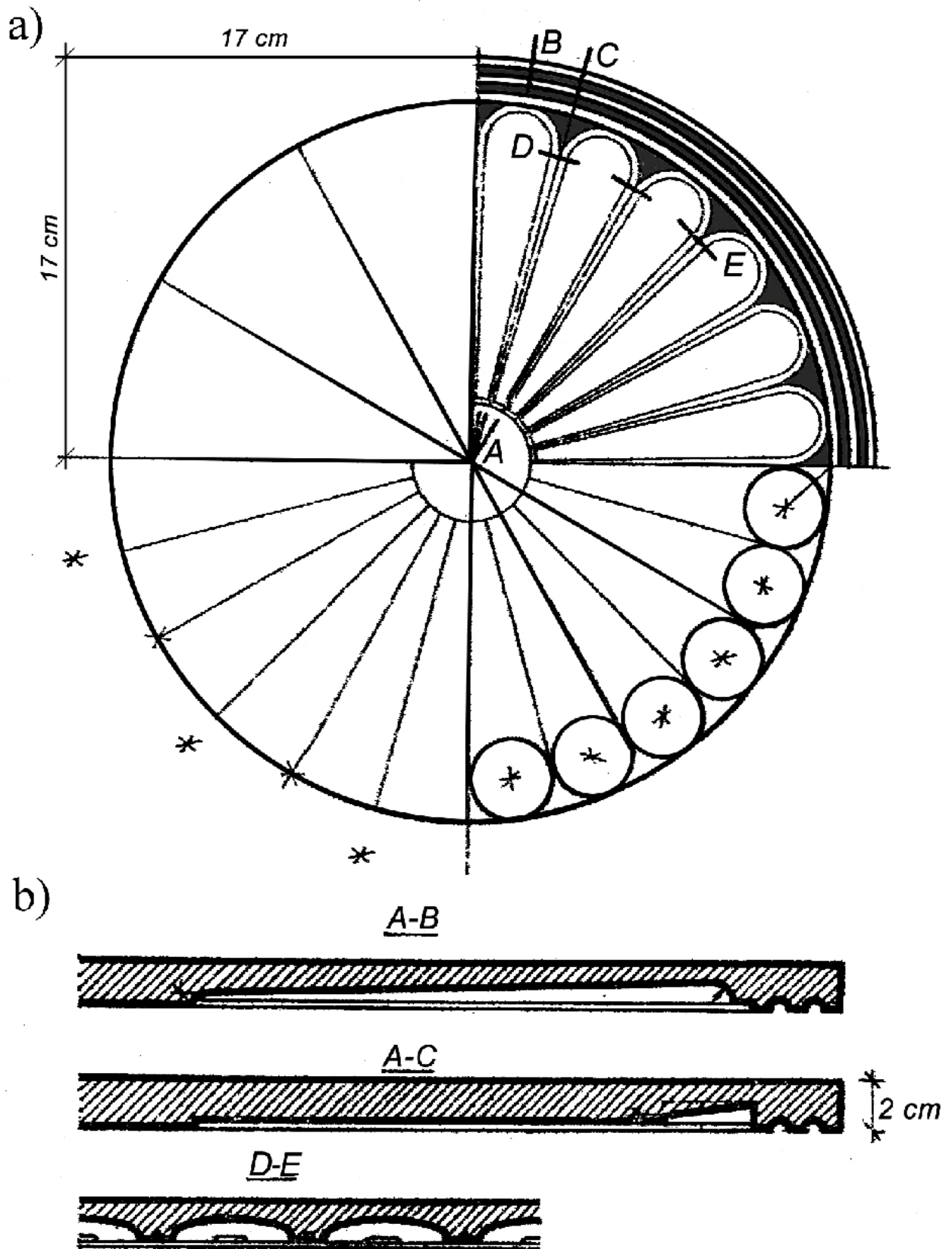
Rysunek 2. Rysowanie rozety o układzie promienistym: a) kolejność rysowania, b) przekroje modelu sztukatorskiego
