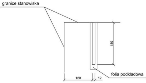
Rysunek 1. Usytuowanie fragmentu ścianki działowej na stanowisku
