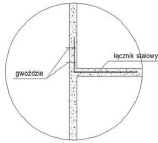
Rysunek 2. Widok lica ściany
