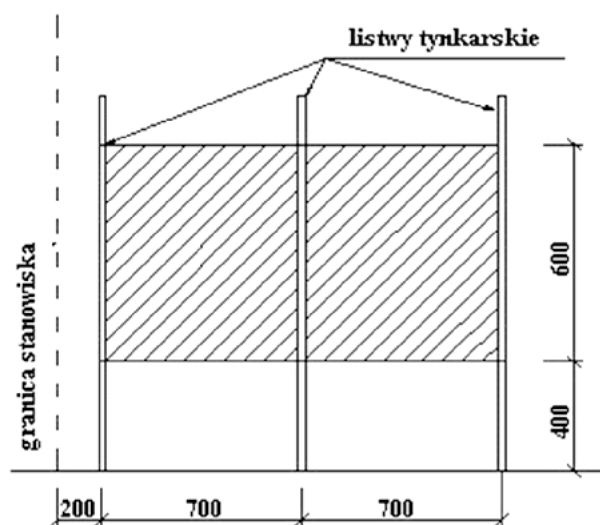
Rysunek 2. Widok ściany przeznaczonej do wykonania narztu
