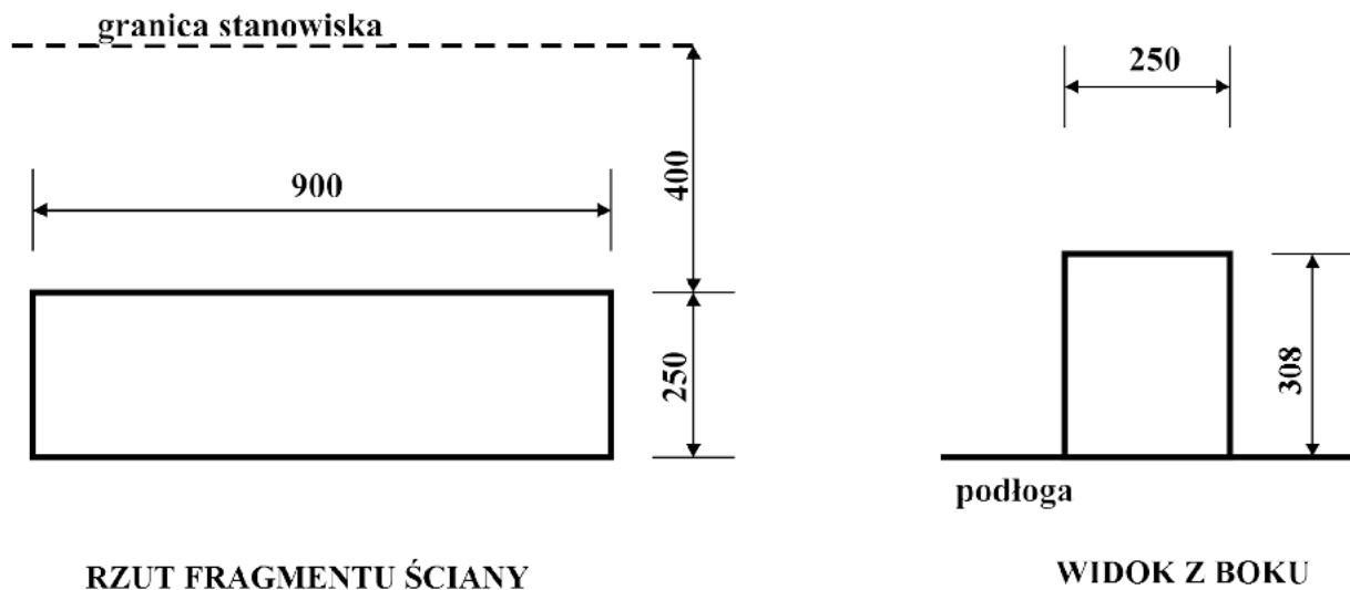
Rysunek 1. Widok fragmentu ściany do wymurowania
