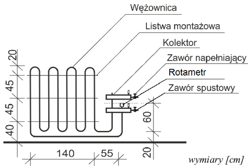
Rysunek. Schemat ogrzewania płaszczyznowego ściennego
