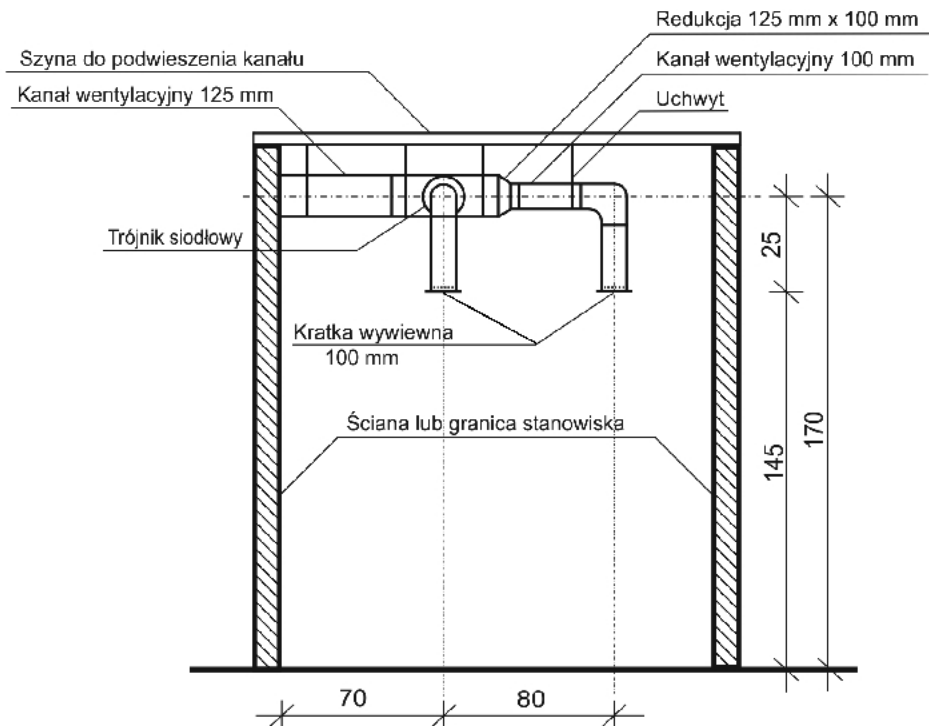
Rysunek 1. Przekrój instalacji wentylacyjnej.
