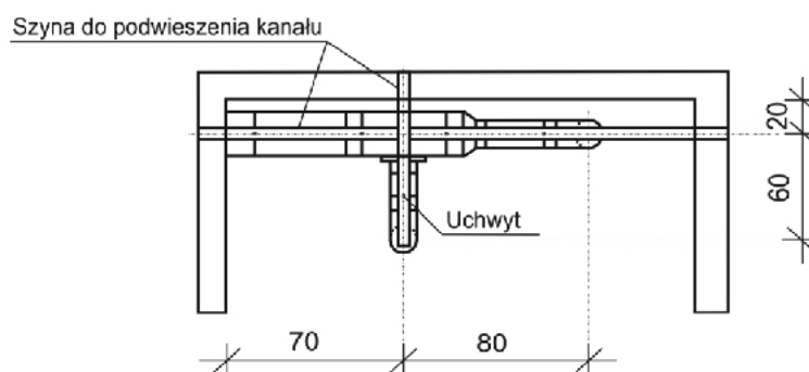
Rysunek 2. Rzut instalacji wentylacyjnej.
