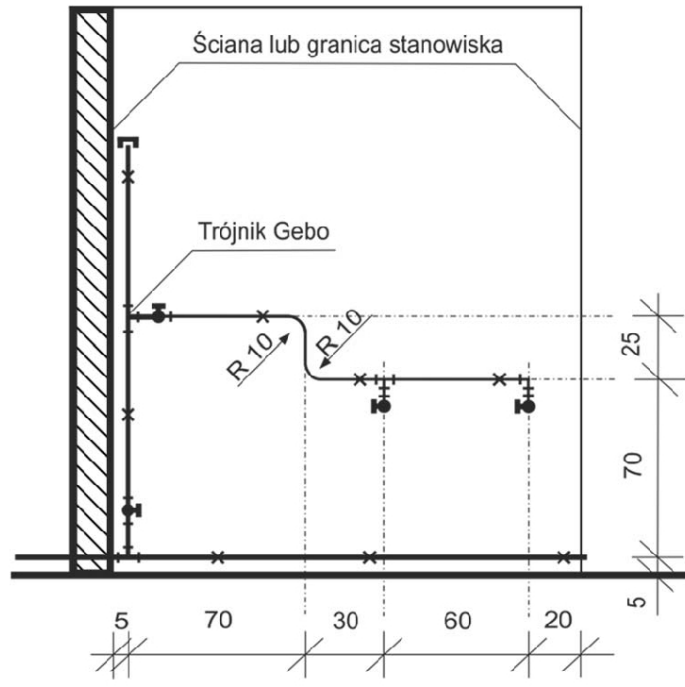
Wymiary podano w cm
