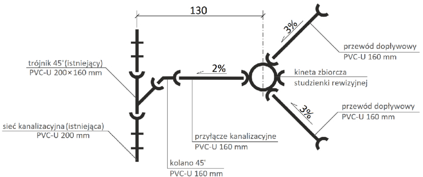
Rysunek. Fragment sieci kanalizacyjnej
