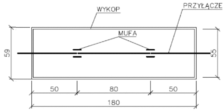
Rzut przyłącza gazowego
