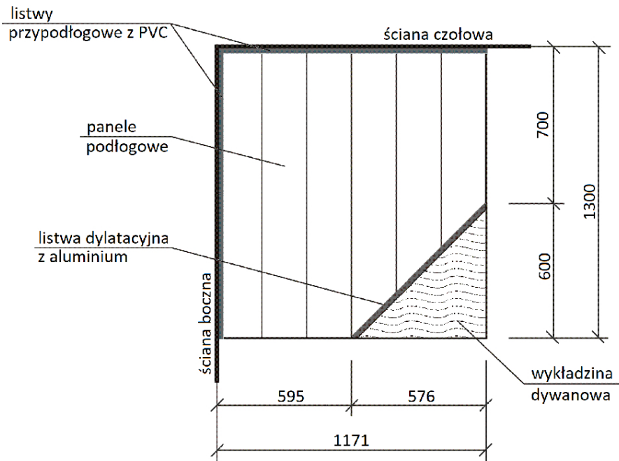
Rysunek. Usytuowanie i układ posadzek – fragment podłogi łączonej Wymiary [mm]
