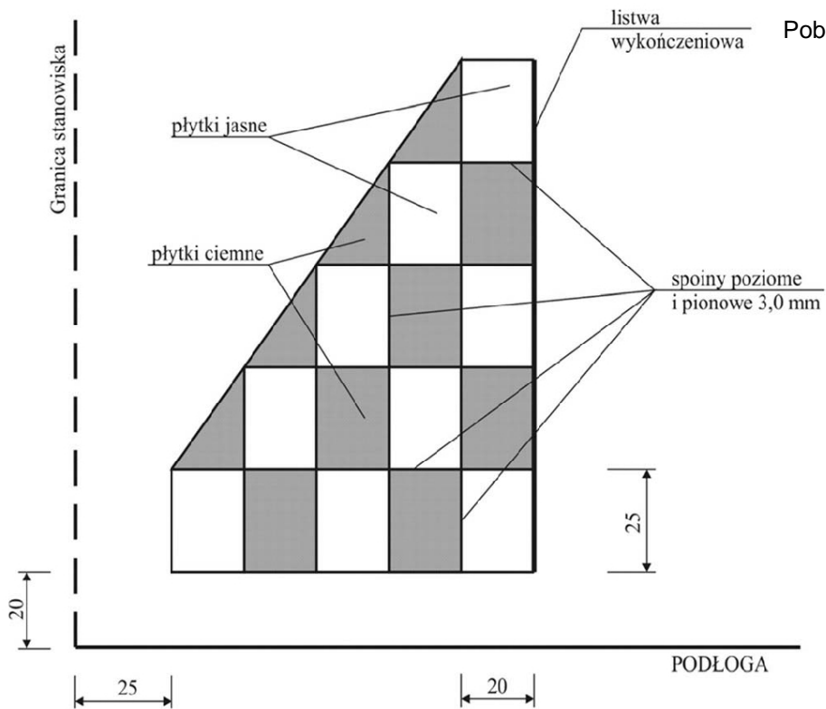
Rys. Widok okładziny ceramicznej
