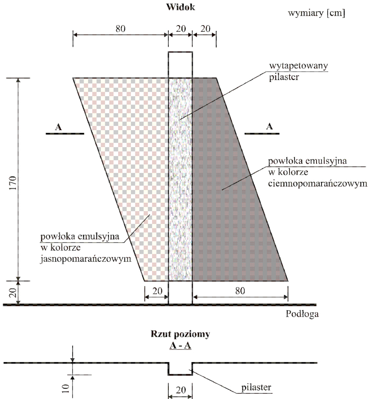
Rys. Widok i rzut poziomy ściany z pilastrem
