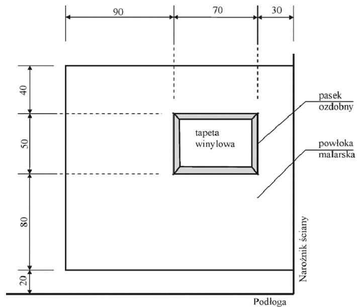
Rys. Widok wykończenia ściany
