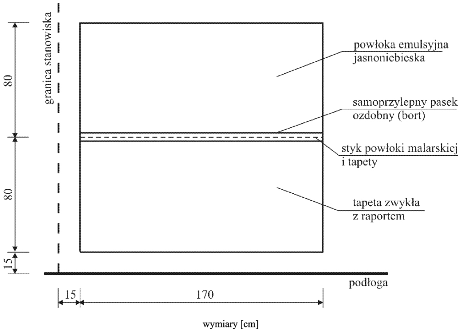
Rysunek 1. Widok wykończenia ściany
