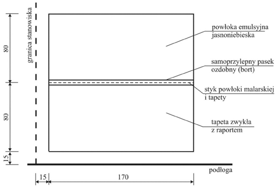
Rysunek 1. Widok wykończenia ściany
