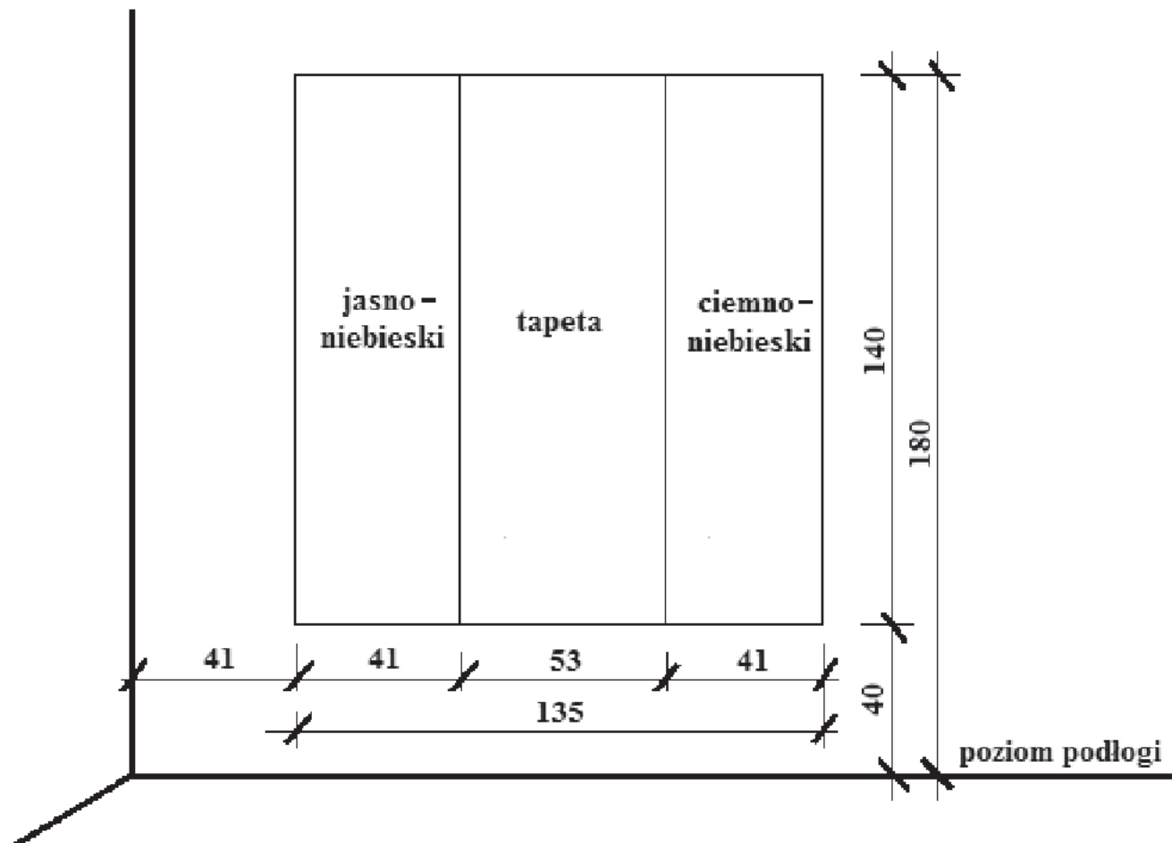
Widok ściany
