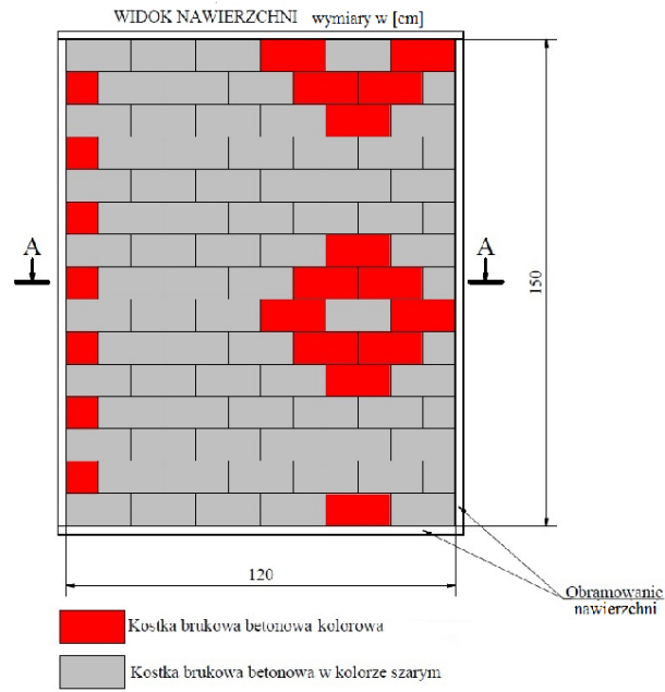
Rys. 1. Rzut poziomy fragmentu nawierzchni do ułożenia
