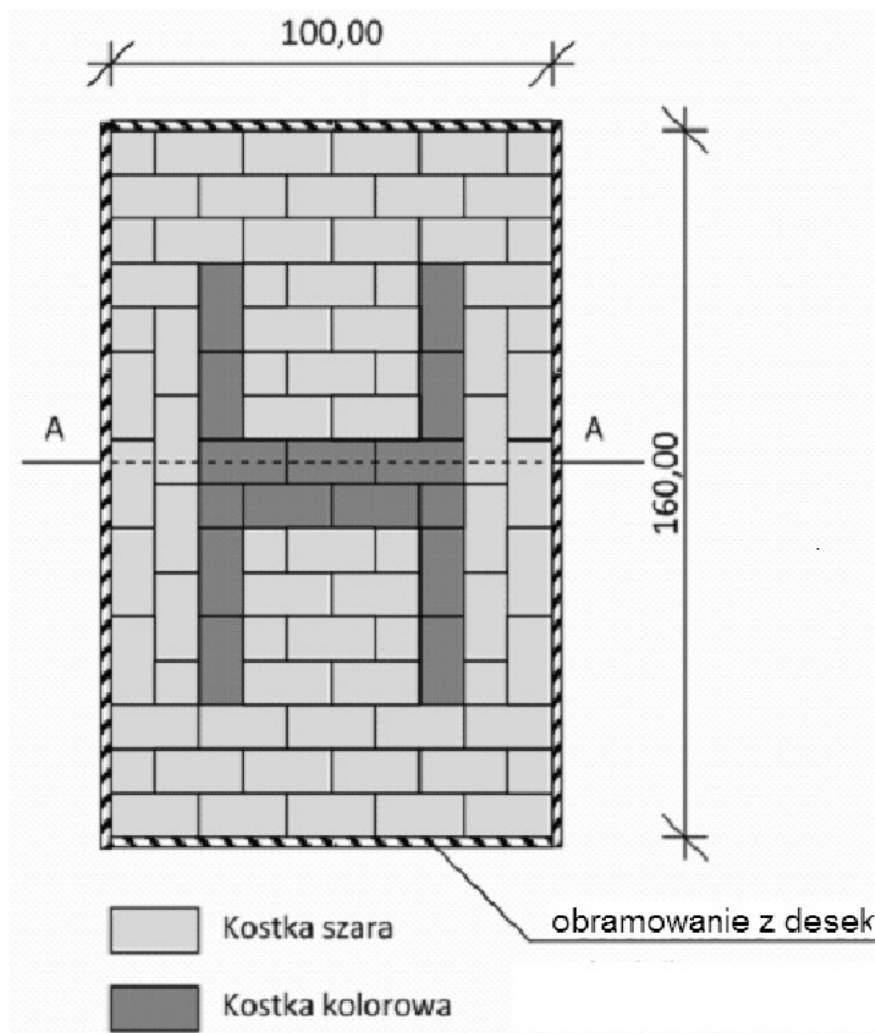
Rysunek 1. Rzut poziomy fragmentu nawierzchni z betonowej kostki brukowej.
