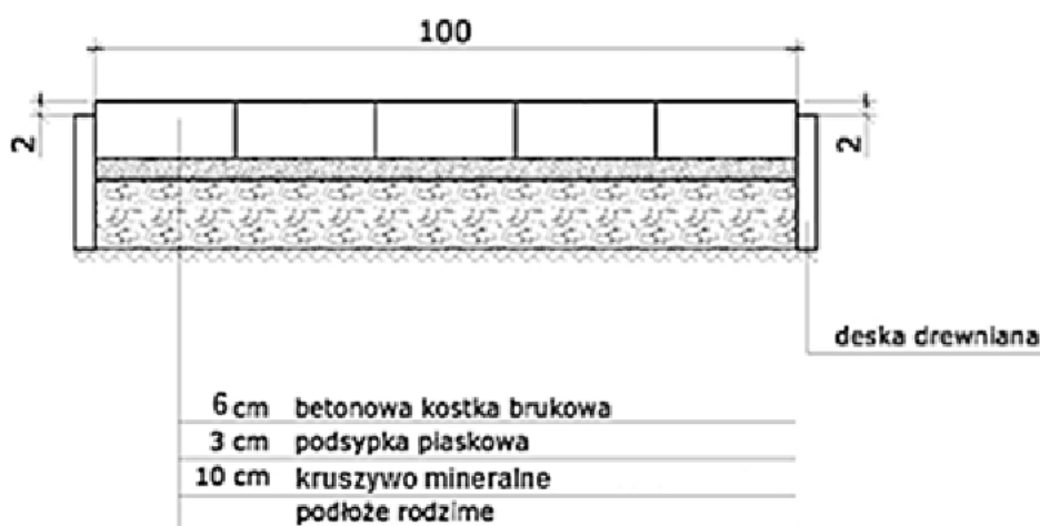
Rysunek 1. Układ kostek betonowych w nawierzchni chodnika
