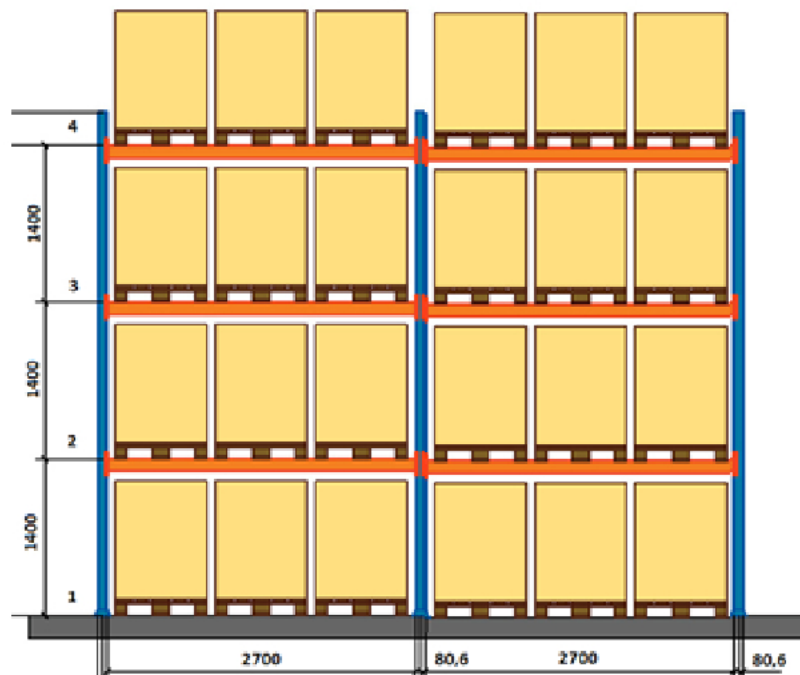
Plan jednego regału magazynowego
