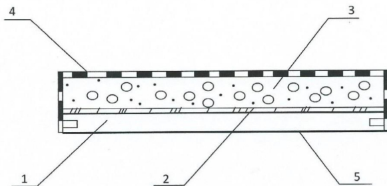
1 - konstrukcja drewniana siedziska; 2 - płyta pilśniowa; 3 - pianka poliuretanowa grubość 80 mm; 4 - tkanina dekoracyjna; 5 - podbitka (tkanina pyłochłonna).
