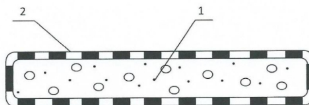
1 - pianka poliuretanowa 400×400×60 mm; 2 - tkanina dekoracyjna.
