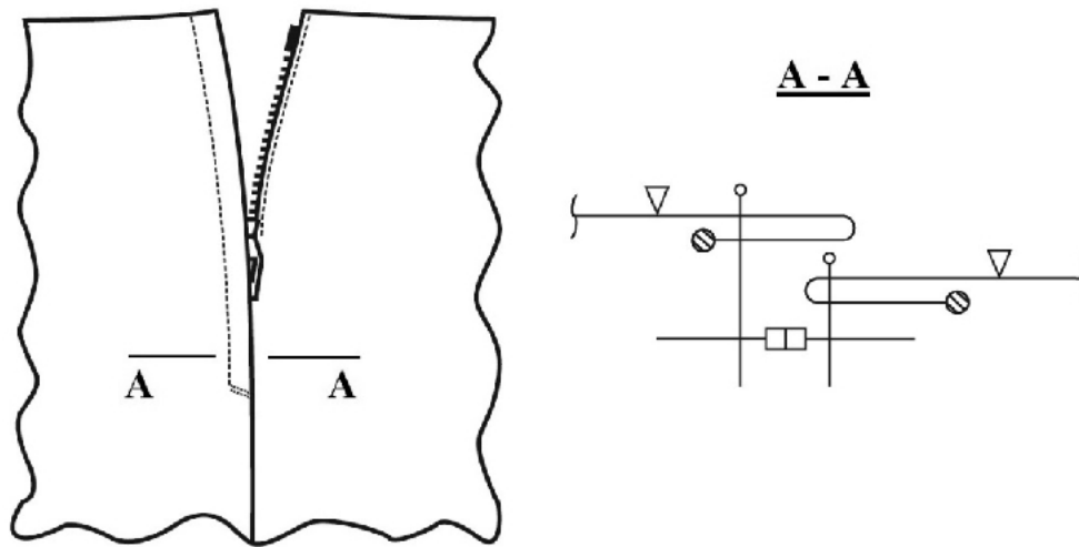
Rysunek 2. Rysunek instruktażowy – wszycie zamka do spódnicy
