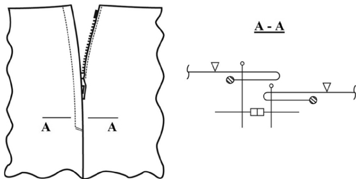
Rysunek 2. Rysunek instruktażowy – wszycie zamka do spódnicy
