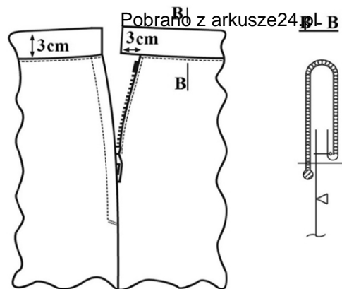
Rysunek 3. Rysunek instruktażowy – wszycie paska do spódnicy
