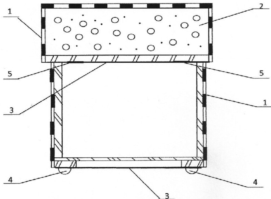
Rys. 1 – przekrój pufu
